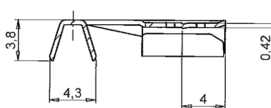
Sez. A-A
