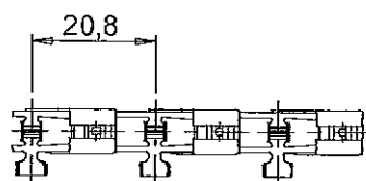
Sez. A-A
