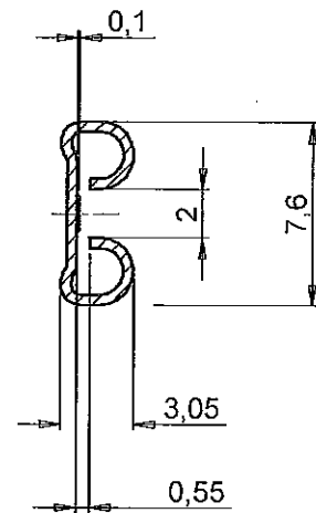
Sez. B-B
